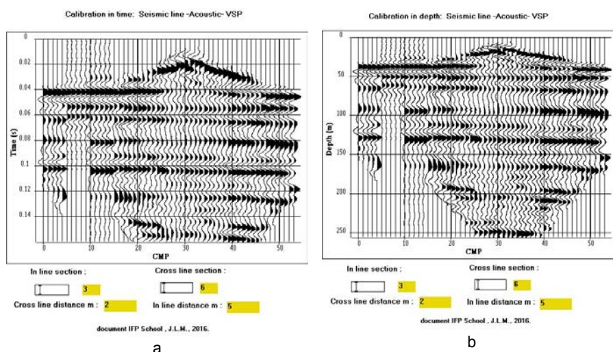
Figure 4.9 Calage d'une section sismique à l'aide d'un PSV et d'une diagrapie acoustique. a : en temps, b : en profondeur.
