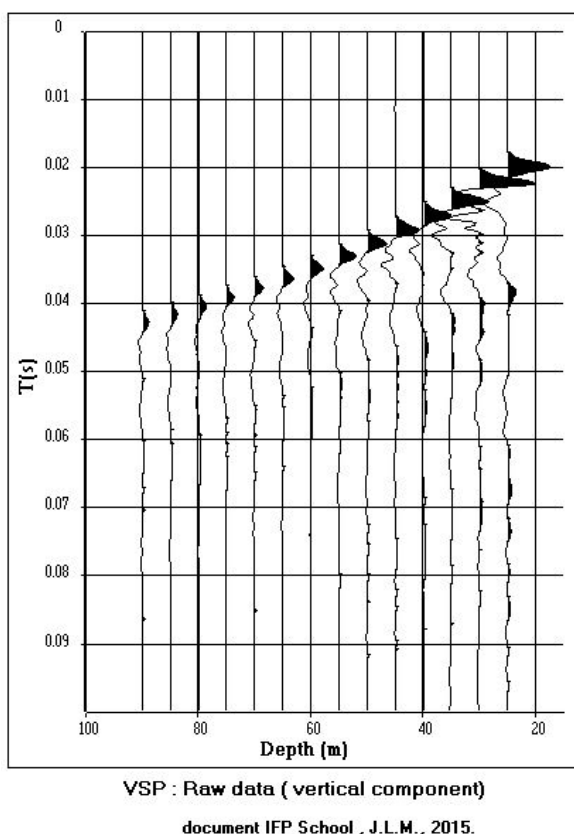
Figure 2.1 Exemple de PSV enregistré dans un puits vertical dans l'intervalle de profondeur 25-90 m.
