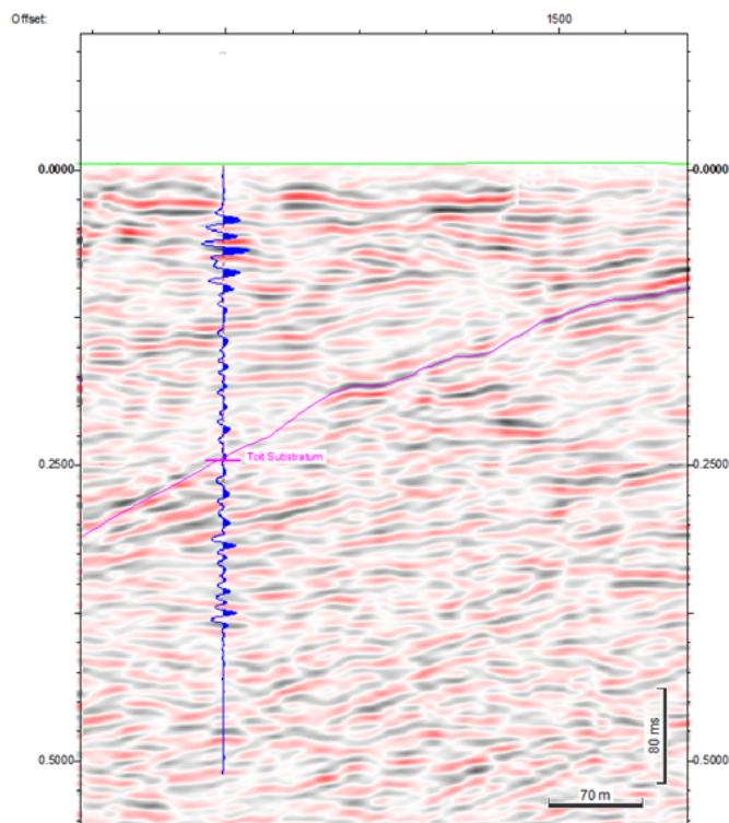
Figure 2.19 Calage d'une section sismique THR sur la trace somme downhole (document : EDF).
