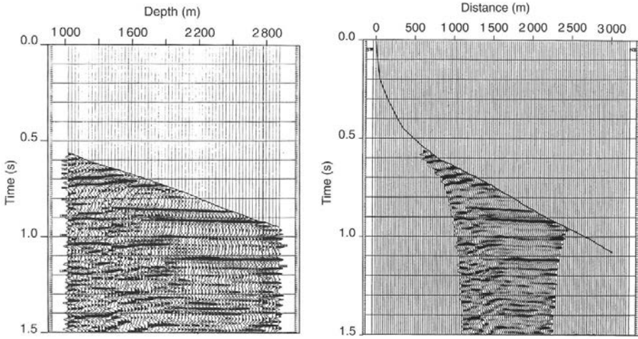
Figure 2.15 PSV en puits dévié (document : BP exploration). À gauche : ondes montantes après déconvolution de Wiener et corrections dynamiques. Lignes d'égale abscisse X (iso-X) présentées tous les 50 m. À droite : section migrée.
