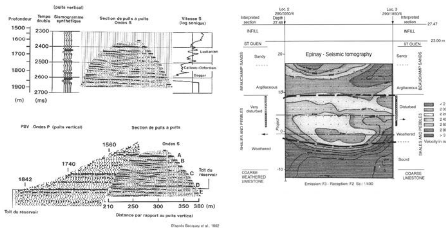
Figure 2.3 Exemples de sismique de puits à puits. À gauche : exemple de sismique de puits à puits en réflexion en ondes S entre un puits vertical et un puits dévié (d'après Becquey et al., 1992). À droite : exemple de tomographie par transmission en génie civil (document : F. Lantier, consultant).
