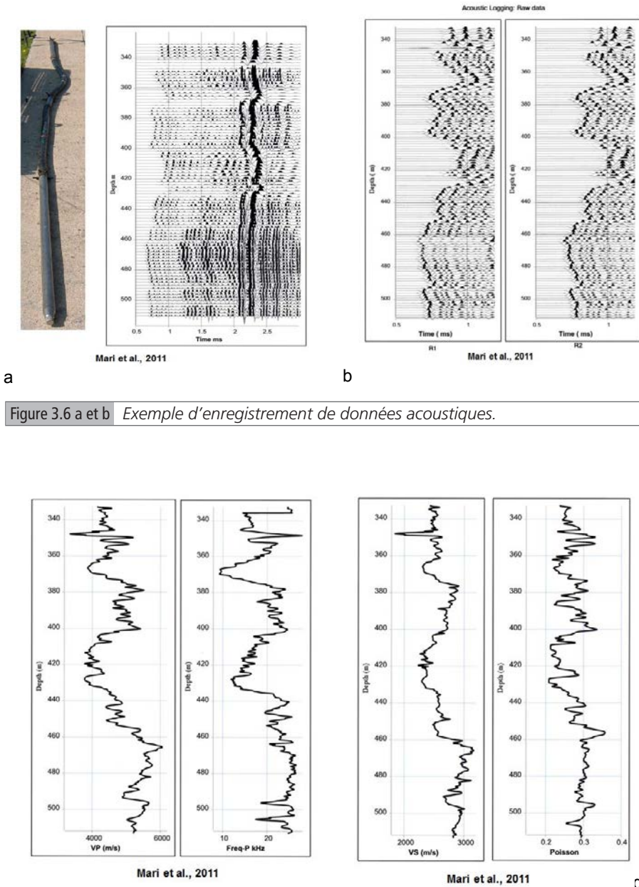
Figure 3.6 a et b Exemple d'enregistrement de données acoustiques. Figure 3.6 c et d Exemple de traitement de données acoustiques – mesure des vitesses. a : outil et section acoustique iso-déport 3m. b : enregistrements acoustiques sur 2 récepteurs séparés de 25 cm. c : logs de vitesse de compression et de fréquence. d : logs de vitesse de cisaillement et coefficient de Poisson.
