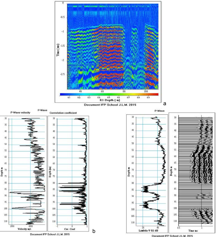
Figure 3.7 Exemple de traitement de données acoustiques. a : section acoustique iso-déport 3m. b : log de vitesse (ondes) et log de corrélation. Les faibles valeurs de vitesse et du coefficient de corrélation indiquent la présence de niveaux karstiques. c : log d'amplitude des ondes P. Les très faibles amplitudes indiquent la présence de niveaux karstiques.
