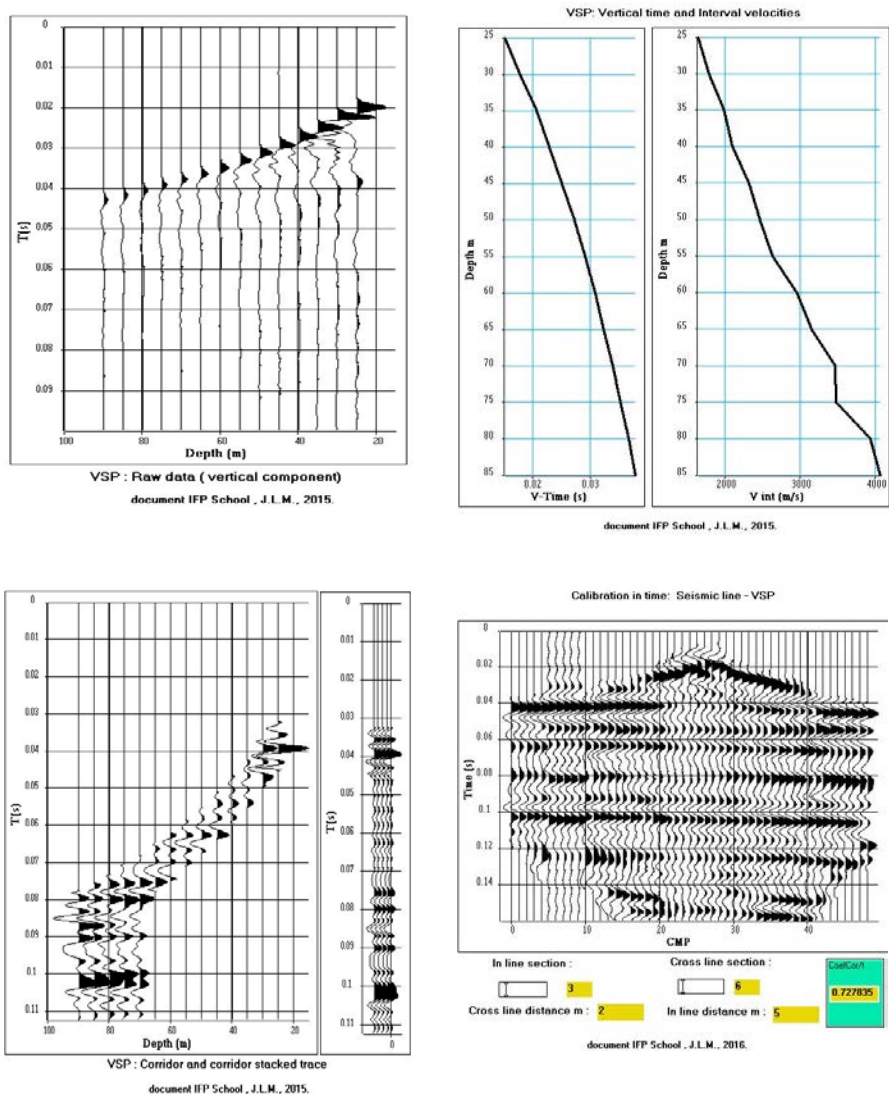
Figure 4.2 Calage d'une section sismique à l'aide d'un PSV.
