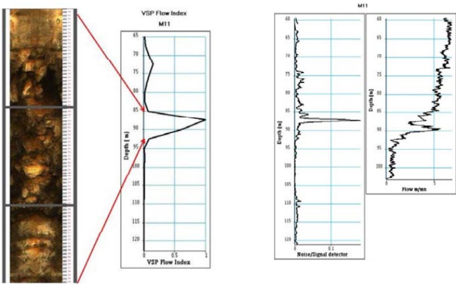
Figure 5.8 Détection de débit dans le forage M11. Comparaison entre imagerie de paroi, indice de flux PSV, détecteur bruit/signal (enregistrement acoustique) et débitmétrie PLT.
