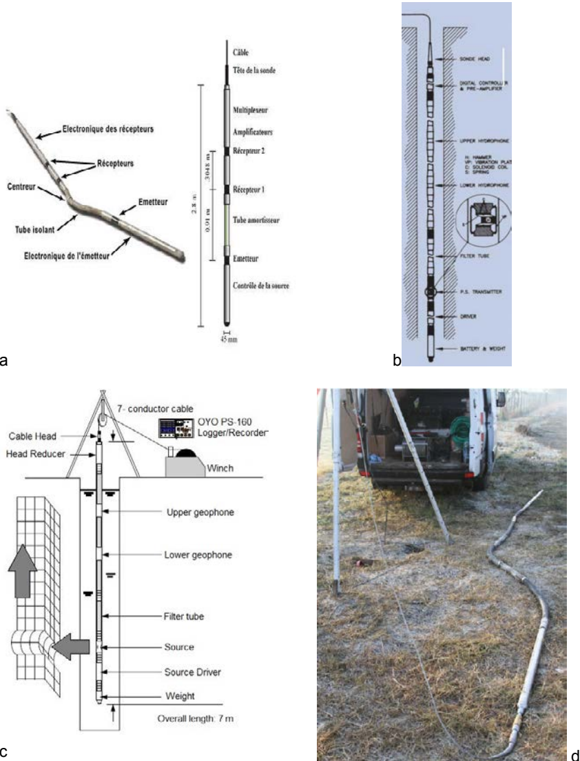
Figure 3.3 Outils acoustiques. a : outil monopôle (Mount Sopris). b : outil dipôle (Robertson). c et d : PSSS (OYO) principe et vue de l'outil (document : GeoVision-EDF).
