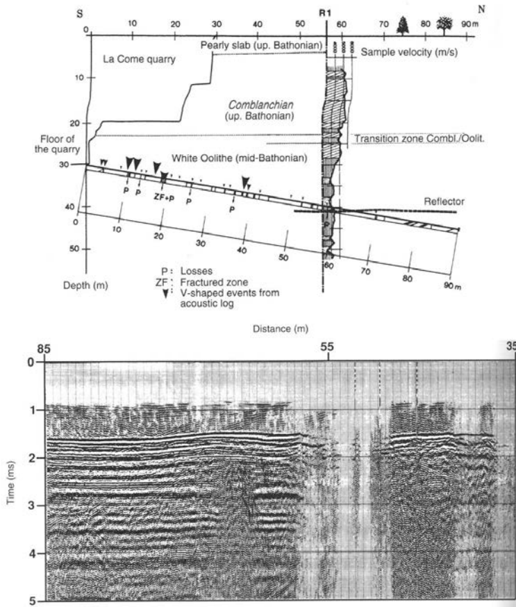
Figure 3.11 Imagerie acoustique en carrière (d'après Mari et al., 1994). En haut : coupe géologique de la carrière de Ravières. En bas : section acoustique à déport constant (3 m). Données brutes.
