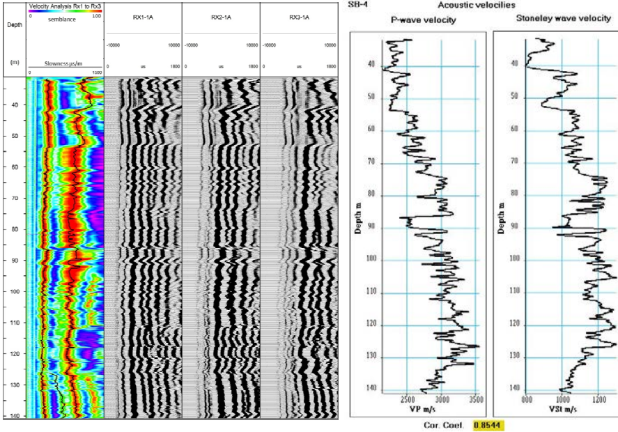
Figure 3.14 Diagraphie acoustique en formation lente. À gauche : panneau de vitesse et sections acoustiques à départ constants. À droite : logs de vitesse des ondes P et des ondes de Stoneley.
