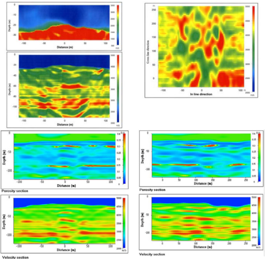
Figure 5.3 Traitement sismique 3D. En haut à gauche : inline 31 section de pseudo-vitesse (partie supérieure : zoom dans l'intervalle de profondeur 0-35 m). En haut à droite : carte pseudo-vitesse à 87 m de profondeur. En bas à gauche : inline 21 section en pseudo-vitesse et porosité. En bas à droite : crossline 24 section en pseudo-vitesse et porosité.
