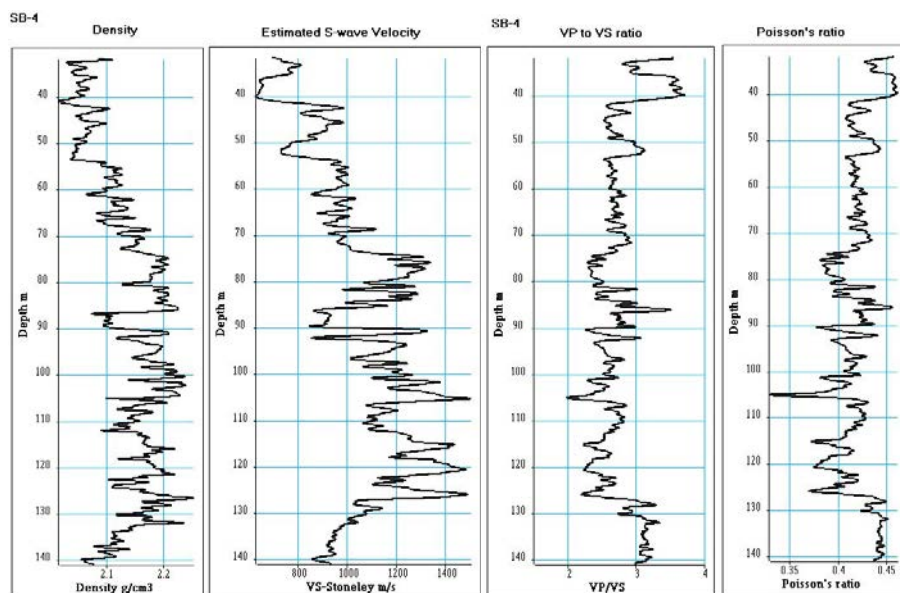
Figure 3.15 Logs acoustiques, de gauche à droite : densité, vitesse S estimée par la vitesse des ondes de Stoneley, rapport V_p sur V_s et coefficient de Poisson.
