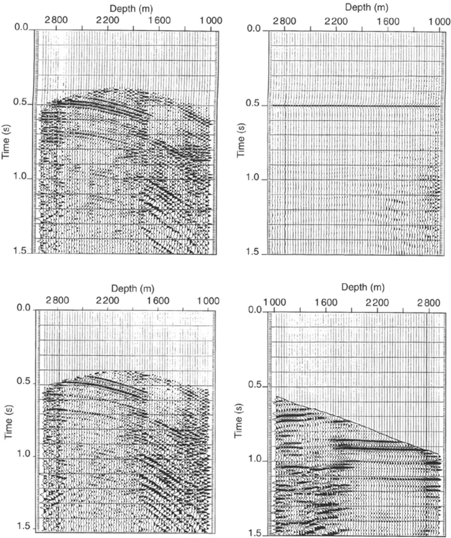
Figure 2.14 PSV en puits dévié (document : BP exploration). En haut : section PSV résidu et ondes descendantes déconvoluées. En bas : ondes montantes après déconvolution et après corrections dynamiques.
