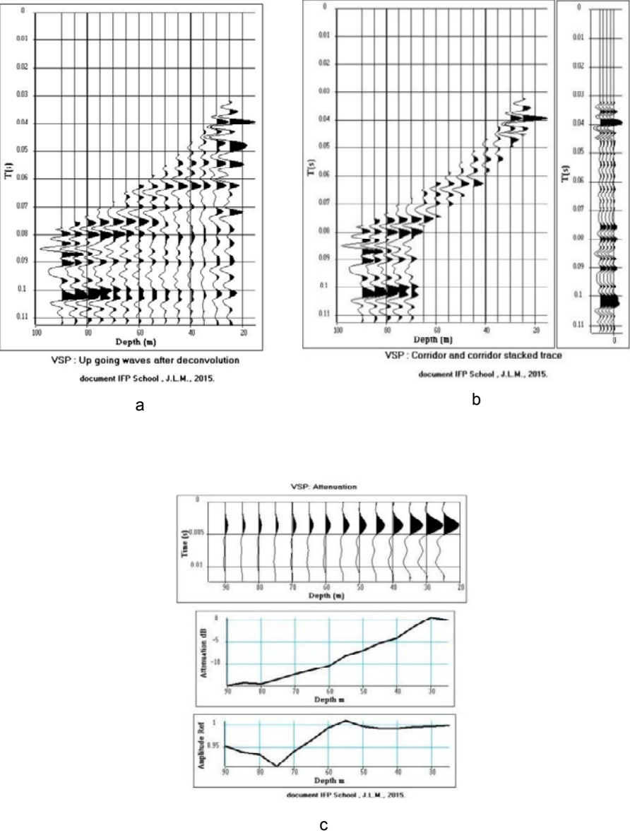
Figure 2.12 Traitement d'un PSV de proche surface. a : ondes montantes déconvoluées. b : couloir de sommation et trace somme. c : mesure d'atténuation (traces PSV, log d'atténuation, référence).
