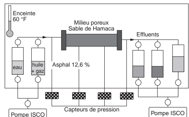
Massif L = 0.5 m ; \Phi = 0.36 ; K = 16.4 °F ; Vitesse de production 0,011 cm 3 /min Slim tube L = 6,1 m ; \Phi = 0,33 ; K = 14 D ; Vitesse 0,001 cm 3 /min
