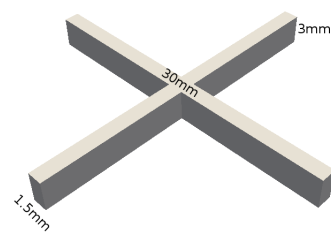
(b) DEM shape
