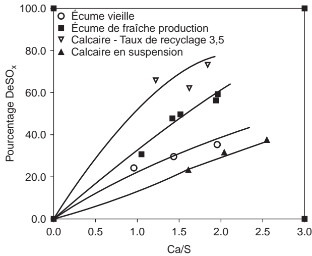
Figure 11 Désulfuration sur chaudière semi-industrielle. Desulfurization in a semi industrial boiler.
