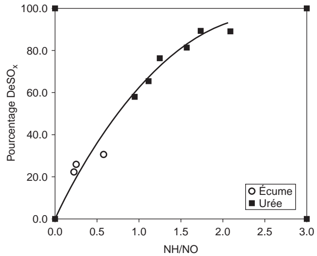
Figure 12 Réduction des oxydes d'azote par l'écume de sucrerie Carbonatation line effect on NO x reduction.
