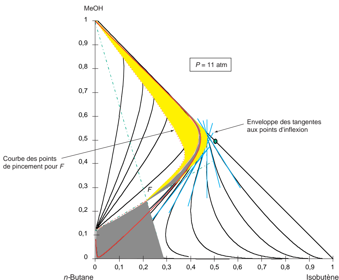
Figure 20 Faisabilité à reflux fini : domaines de produits pour une alimentation dans le champ supérieur (dépassement de la barrière de distillation). Feasible products concentration regions for a finite reflux ratio distillation of a feed mixture located in the superior zone.
