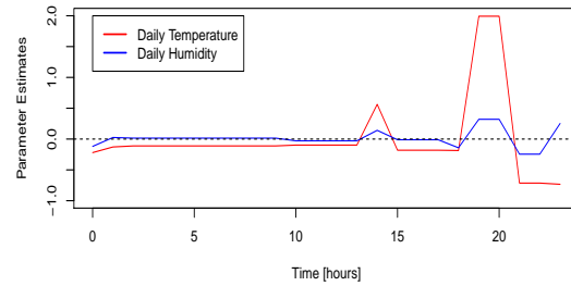
(d) Adaptive fused group quantile solution
